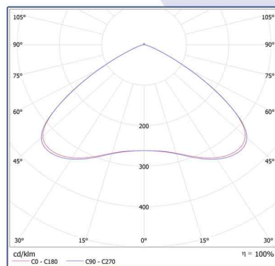
Campana LED 200W Óptica 120°
